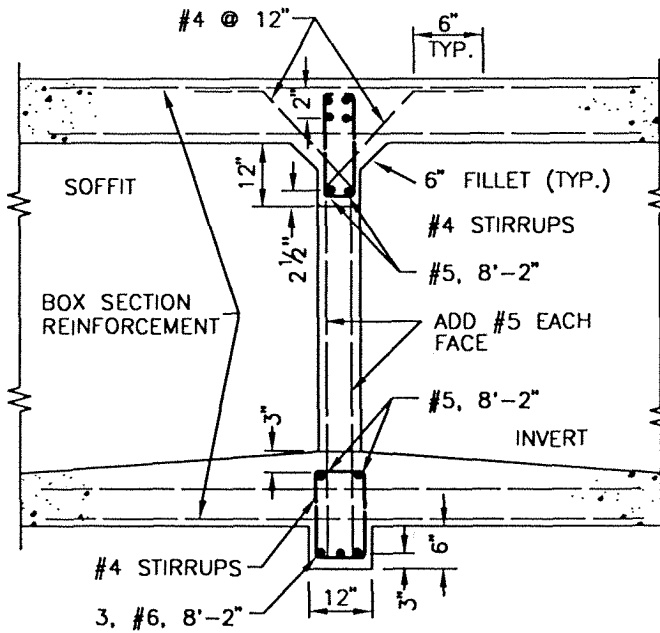
SECTION A-A
