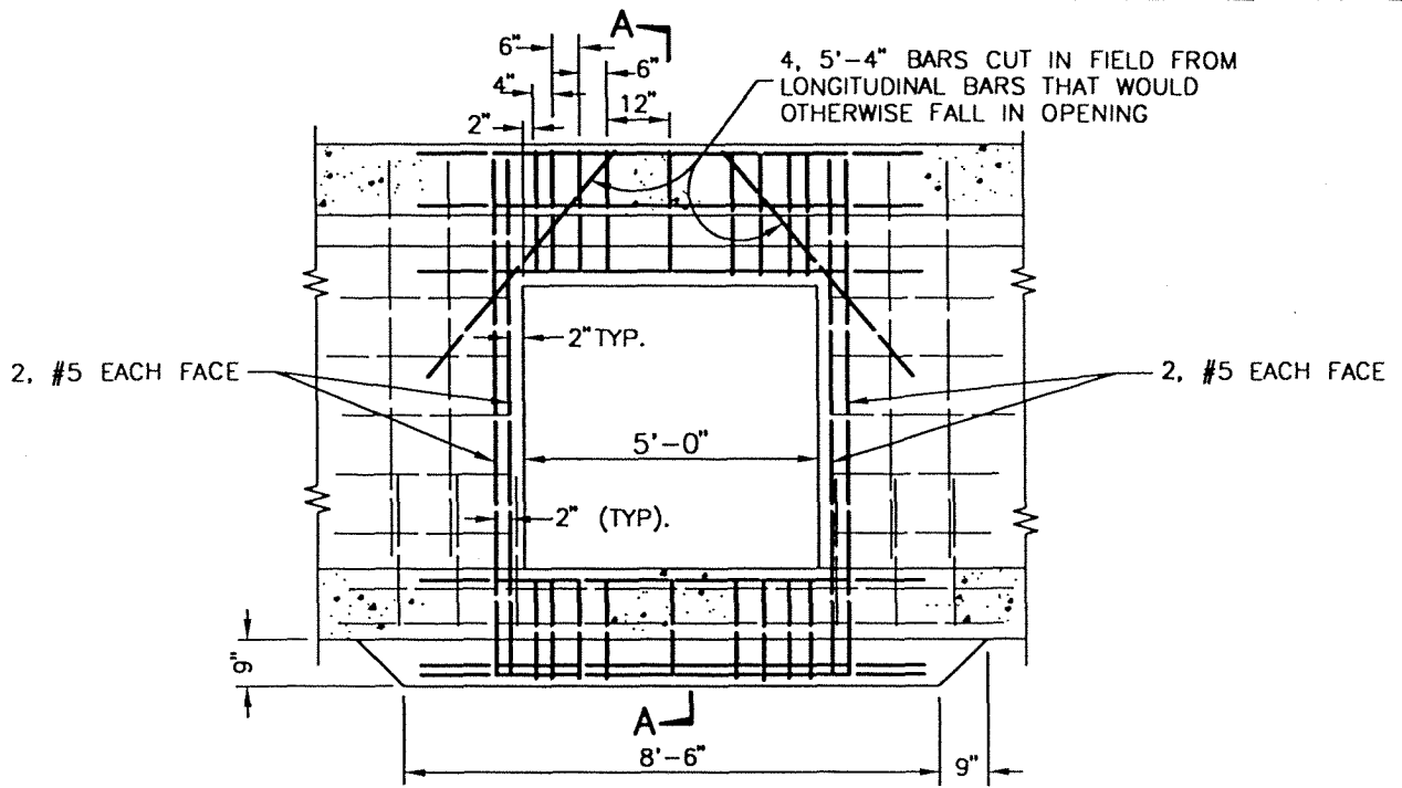
ELEVATION
